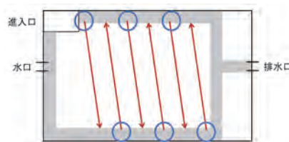
図2＝暗渠施工例
