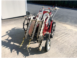
たまねぎ掘取機
