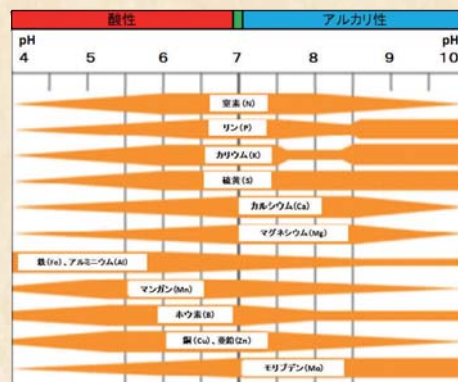
土壌のpHと主要な肥料成分の溶解度 (農林水産省資料より抜粋)
